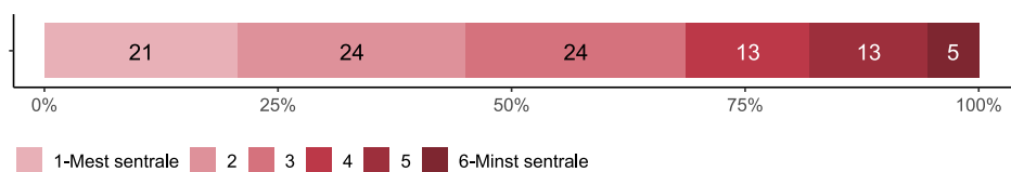
Figure 2: Sentralitet.
